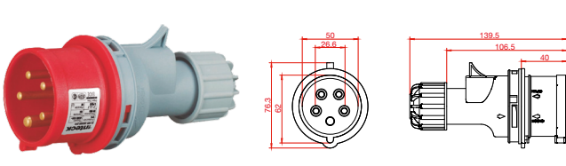
IFI-FM5-16A380V-IP44
