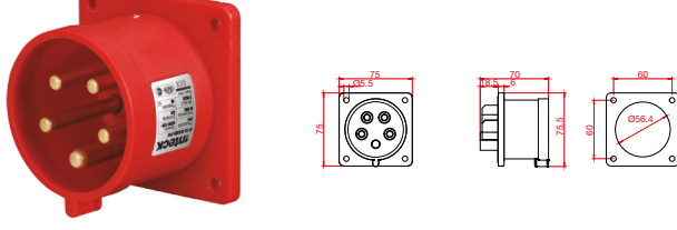
IFI-FE5-32A380V-IP44
