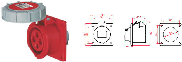
IFI-TE4-63A380V-IP67
