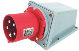
IFI-FS5-63A380V-IP44
