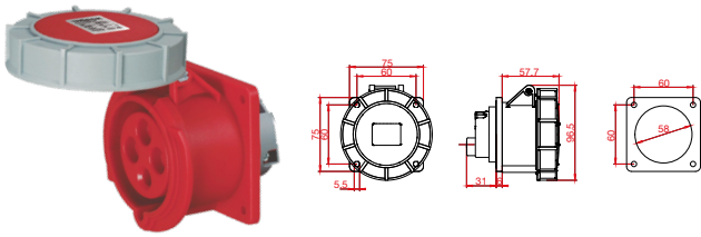
IFI-TE4-32A380V-IP67
