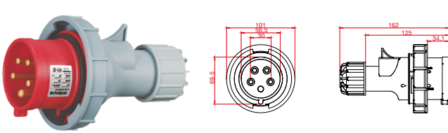
IFI-FM5-32A380V-IP67
