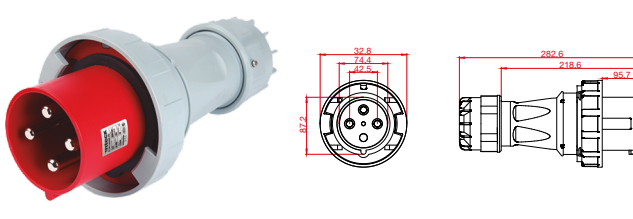
IFI-FM4-125A380V-IP67
