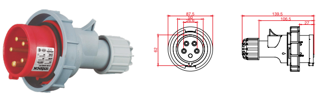
IFI-FM5-63A380V-IP67
