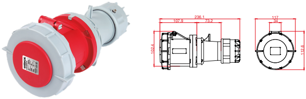
IFI-TM4-63A380V-IP67
