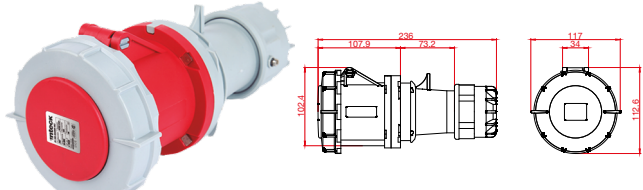
IFI-TM5-63A380V-IP67
