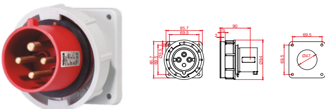
IFI-FE4-32A380V-IP67
