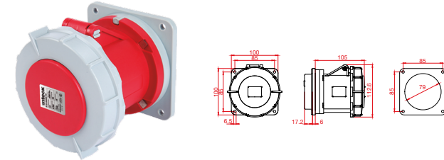
IFI-TE4-63A380V-IP67
