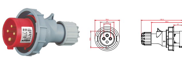
IFI-FM4-16A380V-IP67
